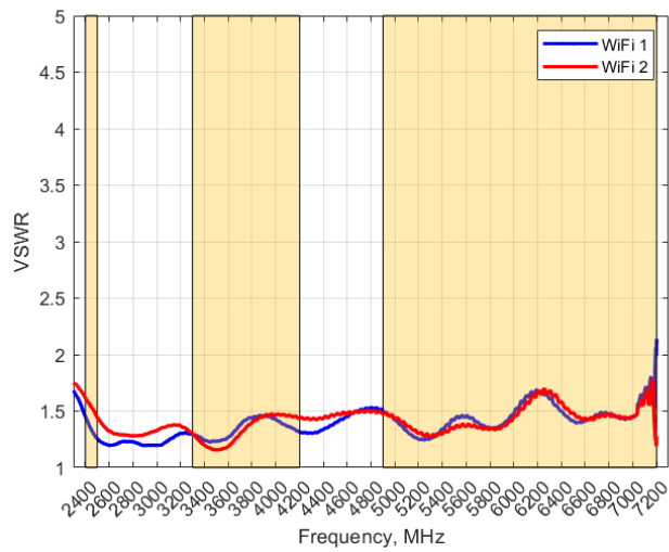
VSWR
