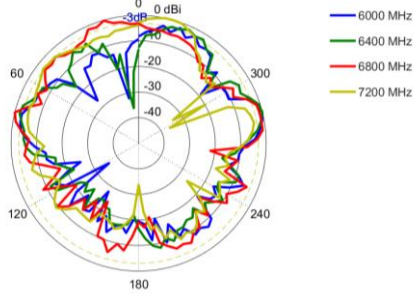
Elevation 2: 6000 – 7200 MHz
